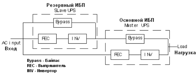
Рис.5-2-1 Система "резервирование Hot-standby"
