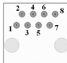
Рис. 3-15: Нумерация выводов интерфейса датчика температуры батарей
