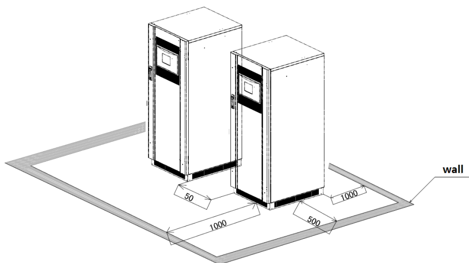
Рис. 3-3: Модели 10~40кВА: схема установки [размеры указаны в мм, Wall=стена]
