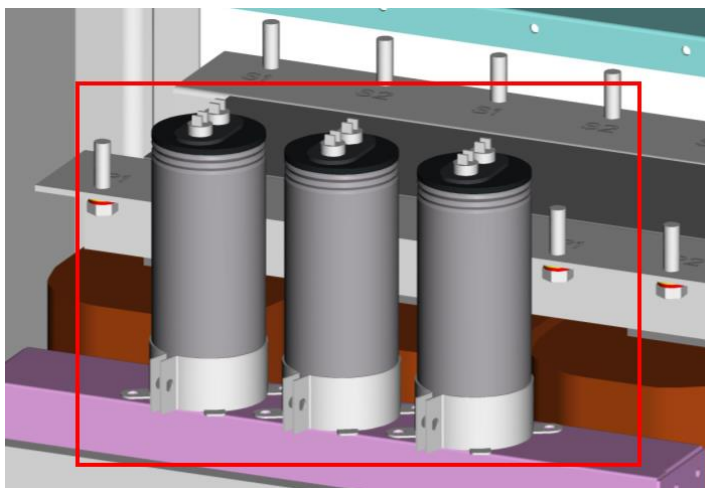
Рис. 2-11: Модели 10~40кВА: Конденсаторы выходного фильтра инвертора (AC output module)
