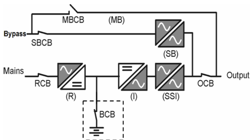
Рис. 2-1: Функциональная блок-диаграмма одиночного ИБП
